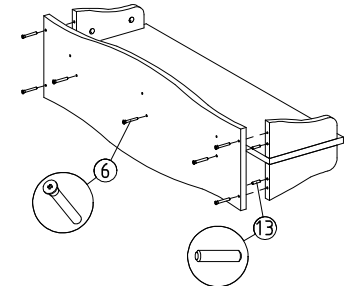
⑥ Tapa minifix montajı
