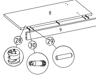
⑬ Sol dikmeye arka perde, alt parça, üst parça ve ön kayıt montajı
