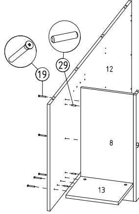
⑫ Arka perdeye alt parça montajı
