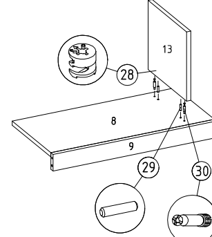
⑭ Sağ dikmeye sağ yan parça montajı
