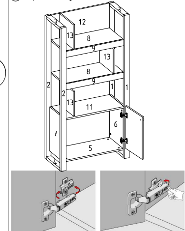
㉑ Kapak montajı
