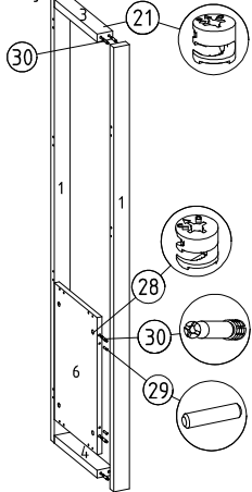
⑯ Sağ yan parça, alt kayıt ve üst kayıt'a sağ dikme montajı
