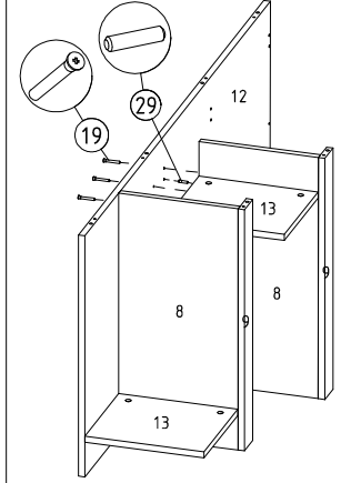
⑮ Sağ dikmeye alt kayıt ve üst kayıt montajı
