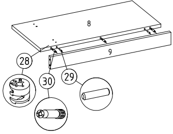
⑩ Üst parçaya dikme montajı
