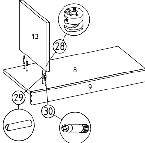
⑪ Arka perdeye üst parça ve dikme montajı
