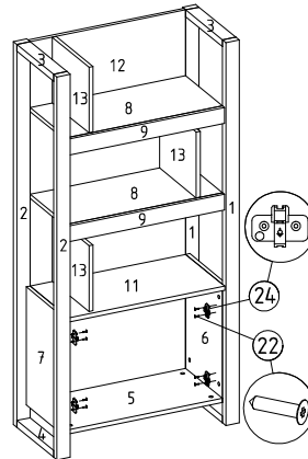
⑱ Mentеше tabanı montajı
