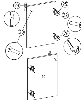
⑲ Kapaklara menteşe ve kulp montajı
