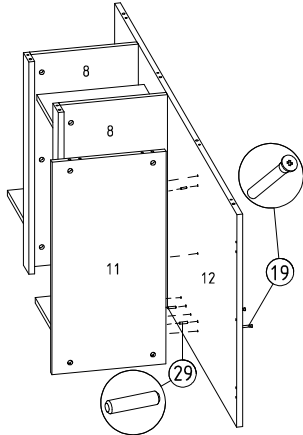
⑰ Arka perde, alt parça, üst parça sabit raf ve ön kayıt'a sağ dikme montajı
