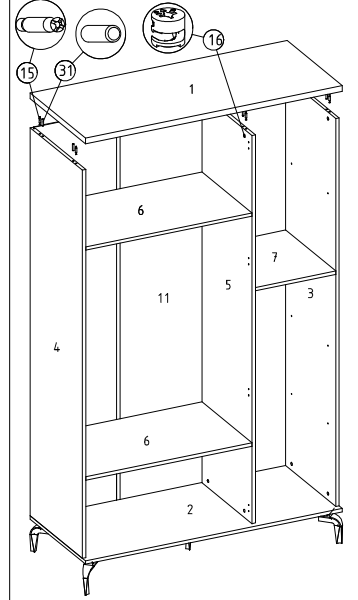
9) Sağ yan parça, sol yan parça ve orta dikmeye üst parça montajı
