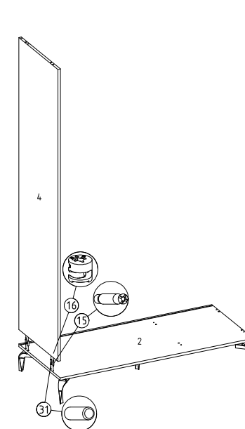
② Alt parçaya sol yan parça montajı
