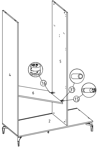
10) Mentеше tabanı montajı
