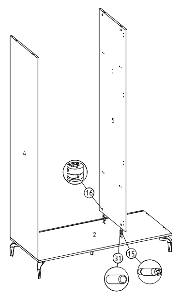
③ Alt parçaya orta dikme montajı
