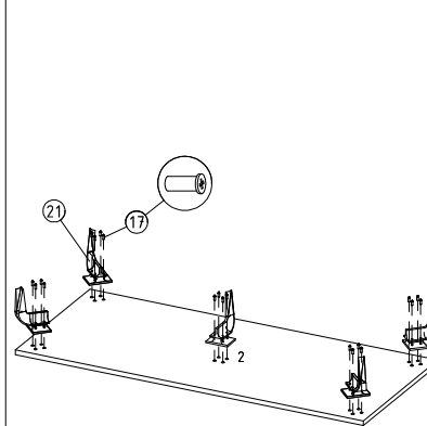
① Alt parçaya ayak montajı
