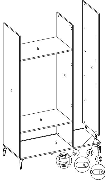
12) Raf pimi montajı
