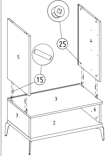
5 Alt modüle sağ sol yan parça montajı
