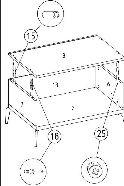
9 Çekmece arka, yan parça ve klapa montajı
