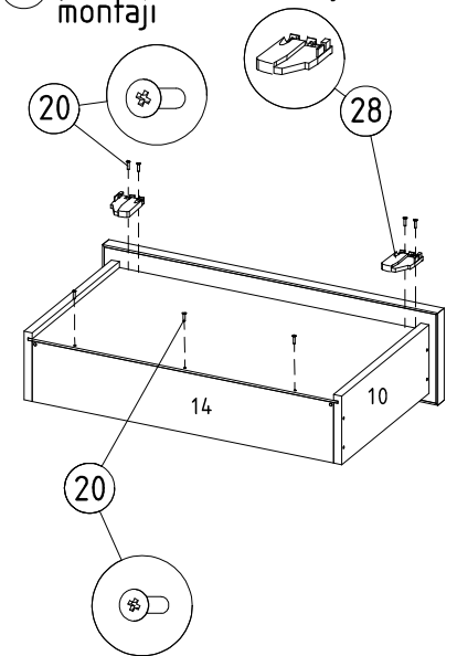
9 Çekmece arka, yan parça ve klapa montajı
