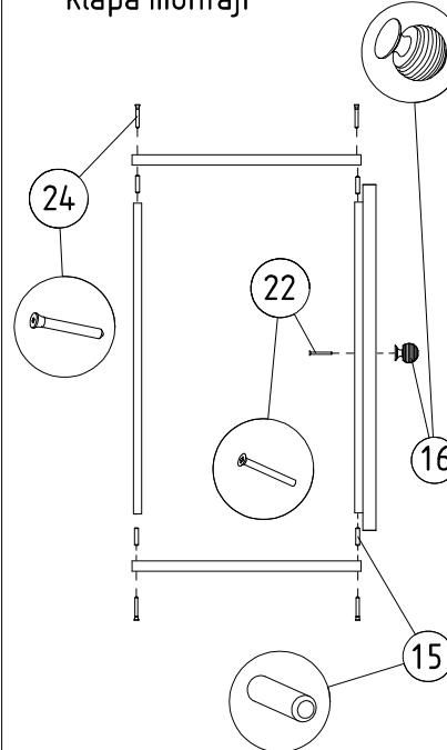
9 Çekmece arka, yan parça ve klapa montajı
