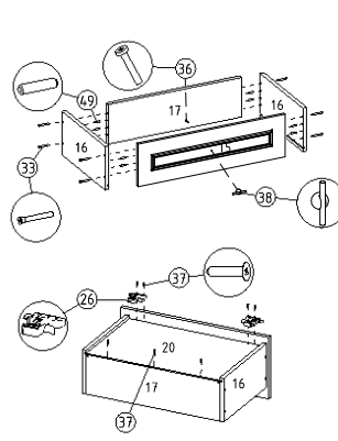
⑮ Çekmece kabini montajı
