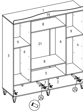
⑲ Raf pimi ve askı flanşları montajı
