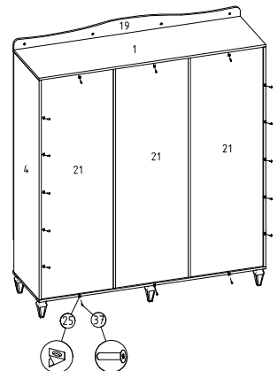
㉑ Arkalık sabitleyici montajı
