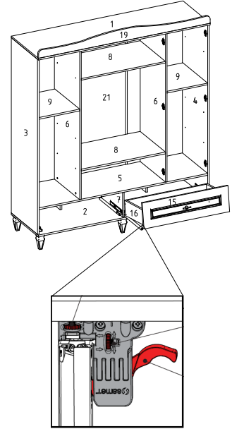
⑯ Çekmece montajı
