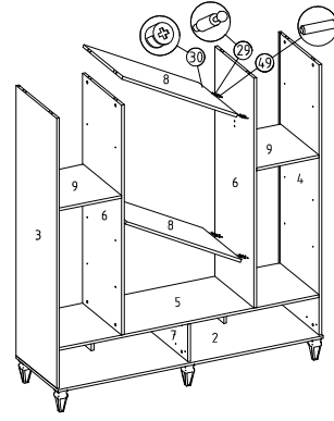
⑮ Çekmece kabini montajı
