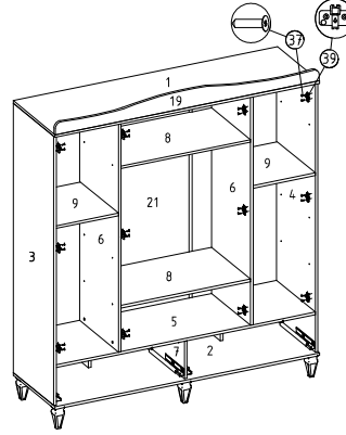
⑭ Mentese tabanı montajı
