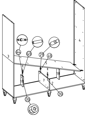
⑫ Sağ yan parça, sol yan parça ve orta dikmeye üst parça montajı
