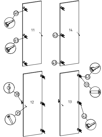
⑰ Kapaklara menteşe ve kulp montajı
