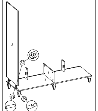
④ Alt parçaya sol yan parça montajı
