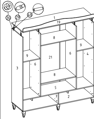
⑫ Sağ yan parça, sol yan parça ve orta dikmeye üst parça montajı
