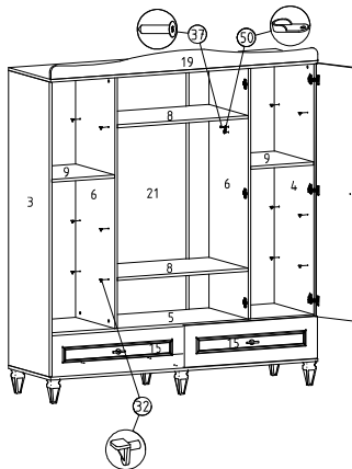
⑲ Raf pimi ve askı flanşları montajı
