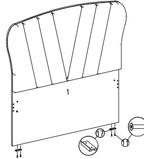
④ Karyola ayak ucuna ayak montajı
