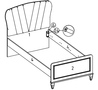
⑥ Galvenizli köşebent montajı
