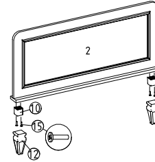
⑦ Karyola demiri montajı
