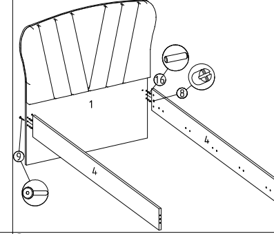
⑤ Travers'e karyola ayak ucu montajı
