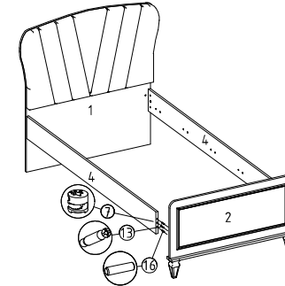
⑧ Yatak altı montajı
