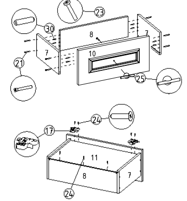
11 Çekmece kabini montajı
