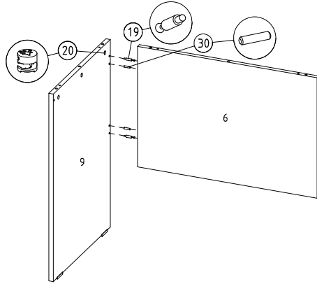
5 Sol yan parçaya arka perde montajı
