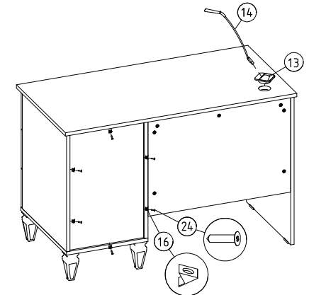
14 Arkalık sabitleyici, şarj cihazı ve okuma lambası montajı
