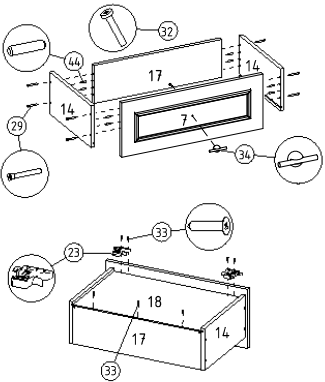
⑯ Çekmece kabini montajı
