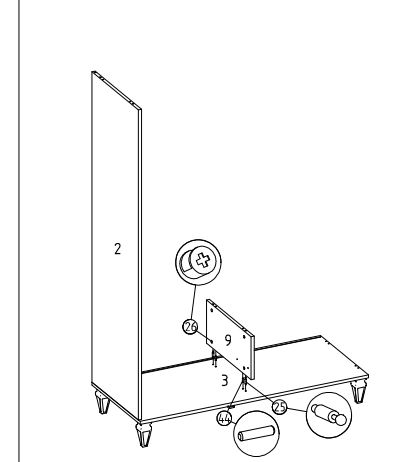
③ Alt parçaya alt dikme montajı
