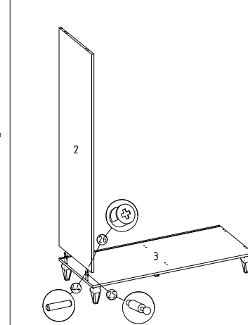
② Alt parçaya sol yan parça montajı
