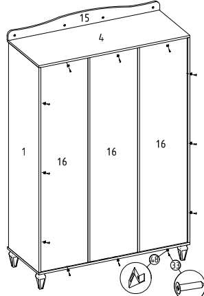
⑱ Arkalıksız abiteyici montajı
