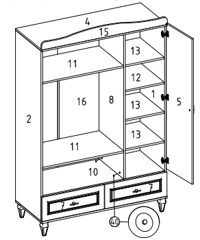
⑳ Kapak ve tapa minifix montajı
