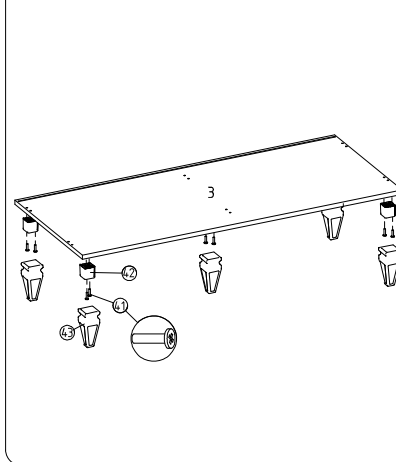
① Alt parçaya ayak montajı
