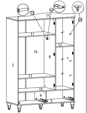
⑳ Kapak ve tapa minifix montajı
