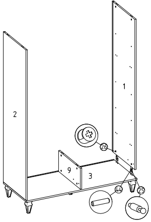
⑩ Arkalık montajı
