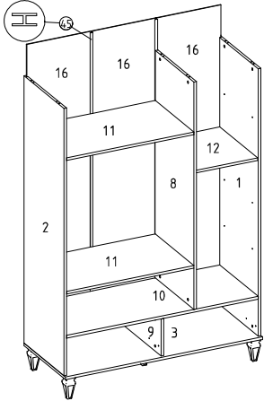
⑯ Çekmece kabini montajı
