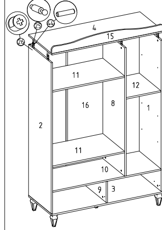
⑫ Sağ yan parça, sol yan parça ve orta dikmeye üst parça montajı
