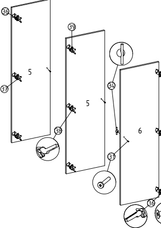
⑲ Kapaklara menteşe ve kulp montajı
