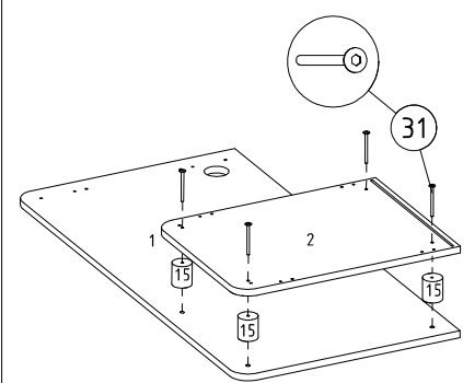
⑨ Üst tablaya modül üst parça montajı
