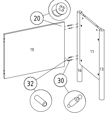
⑦ Sağ arka direğe arka perde montajı
