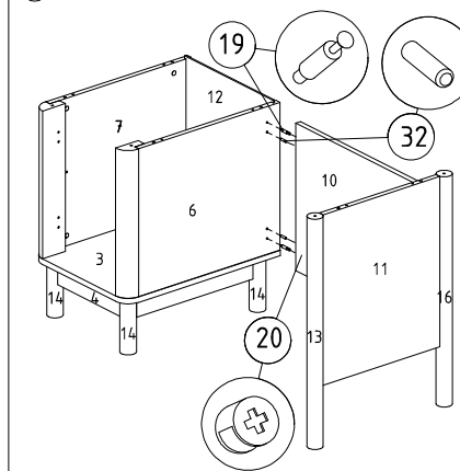
⑧ Modül sağ yan parçaya arka perde montajı
