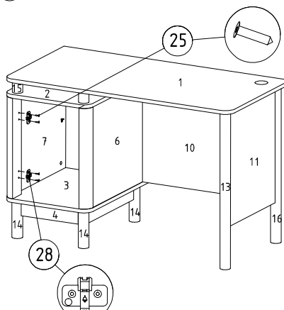
⑫ Menteşe tabanı montajı
