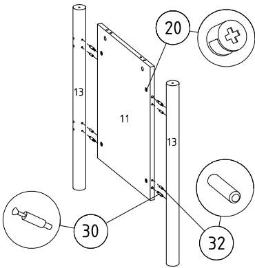
⑪ Raf pimi montajı
