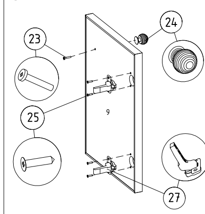
⑬ Menteşe ve kulp montajı
