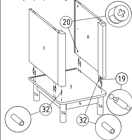
⑨ Üst tablaya modül üst parça montajı
