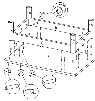
8 Orta parçaya sağ yan parça, sol yan parça montajı
