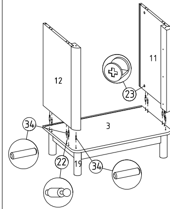
9 Arkalık dar montajı
