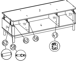
13) Üst parçaya üst kayıt montajı
