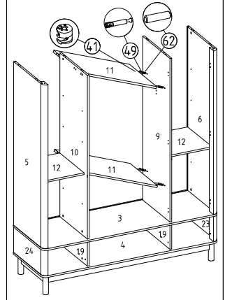
11) Sağ dikme ve sol dikmeye bölme montajı
