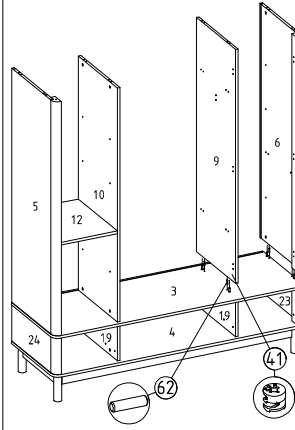
16) Ray montajı
