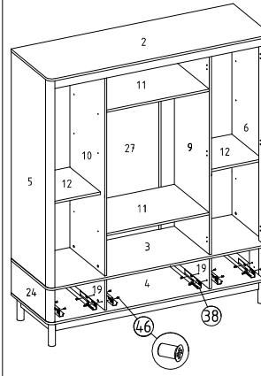
23) Çekmece montajı
