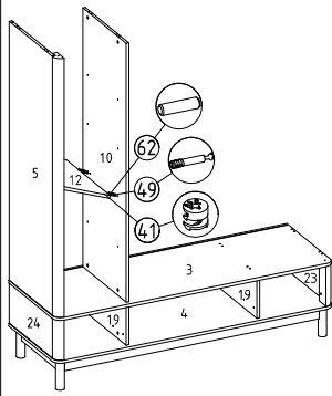
15) Alt sağ parça alt sol parçaya ray destek parçası sağ ve ray destek parçası sol montajı
