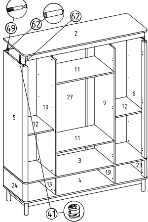
21) Arkalık sabitleyici montajı
