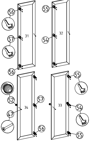
19) Kapaklara menteşe ve kulp montajı
