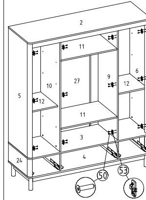
17) Menteşe tabanı montajı
