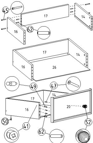
20) Çekme kabini montajı
