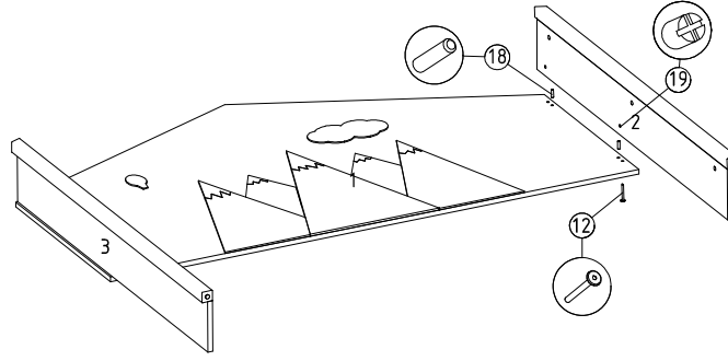
8) Arka parçaya Üst kayıt montajı
