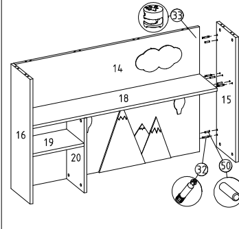
19 Arka kayıta üst dikme montajı
