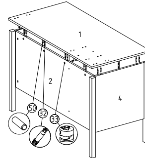
14 Kısa bölmeye sağ dikme ve sol dikme montajı
