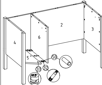
13 Arka parça ve bölmeye sağ yan parça montajı
