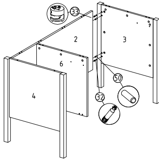
12 Arka parça, bölme ve kısa bölmeye sol yan parça montajı
