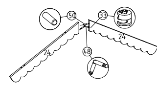
18 Ön kayıt montajı
