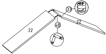
17 Üst dikme montajı
