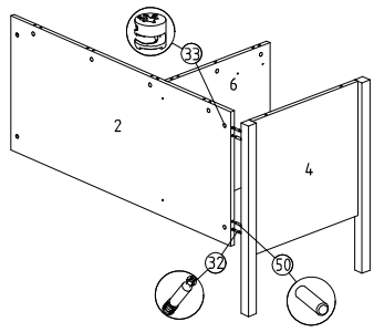
11 Dikmeye kısa bölme montajı
