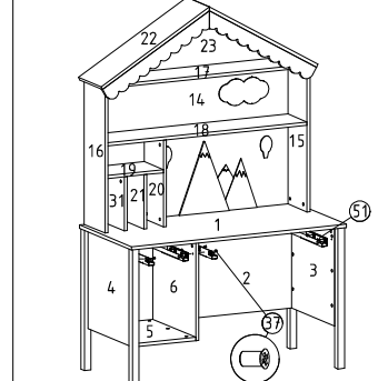
27 Kapak ve tapa minifix montajı
