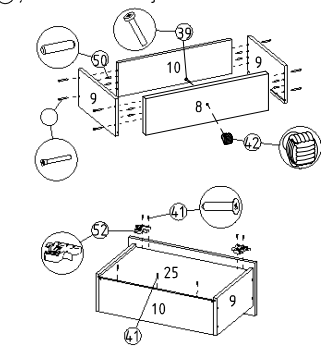
24 Çekmece kabini montajı
