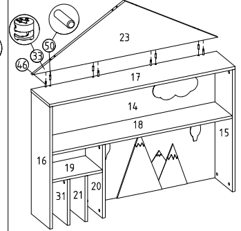
22 Ray montajı
