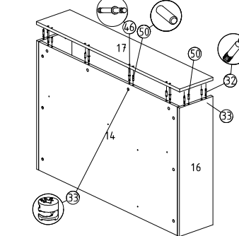
21 Üst tablaya sağ yan parça, sol yan parça, dikme sağ dikme sol dikme montajı
