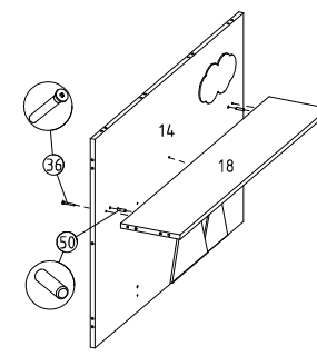
15 Üst parça montajı
