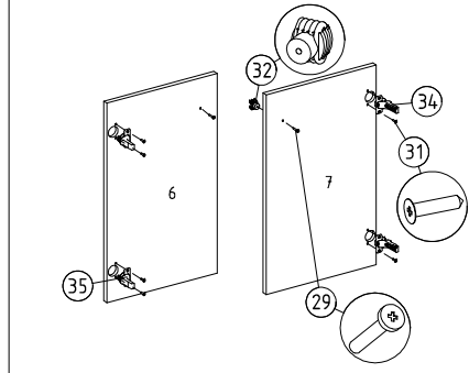
20 Kapaklara menteşe ve kulp montajı
