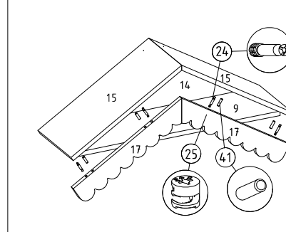
21 Tapa minifix montajı
