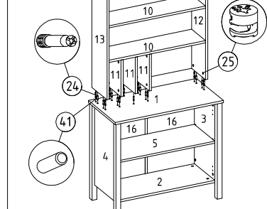
17 Üst tablaya sağ sol yan parça montajı
