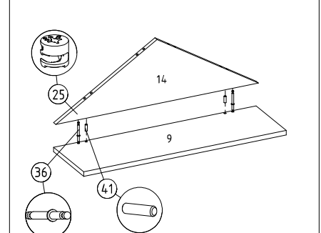
18 Üst parça montajı
