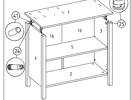
13 Üst parçaya arka kayıt montajı
