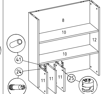
17 Üst tablaya sağ sol yan parça montajı
