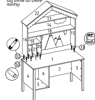
21 Üst tablaya sağ yan parça, sol yan parça, dikme sağ dikme sol dikme montajı
