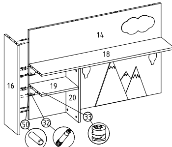
18 Ön kayıt montajı
