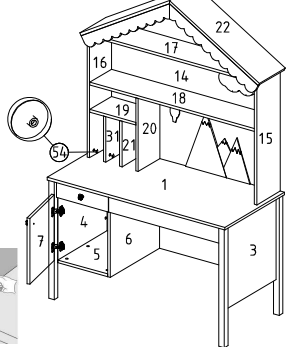
27 Kapak ve tapa minifix montajı
