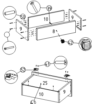
24 Çekme kabini montajı
