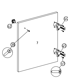
25 Kapağa menteşe ve kulp montajı
