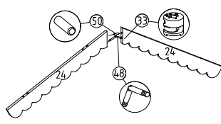
18 Ön kayıt montajı
