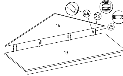
⑫ Üst parçaya arka perde montajı
