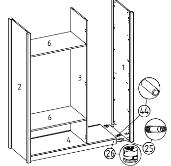
⑬ Ön kayıt montajı
