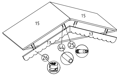
⑳ Arkalık sabitleyici montajı
