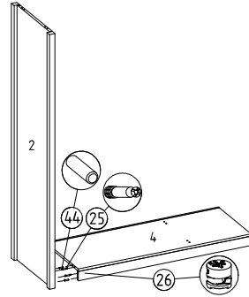
⑩ Arkalık montajı
