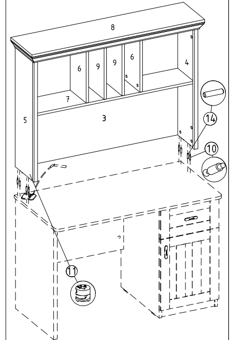
12) Çalışma Masası alta çalışma masası üst montajı
