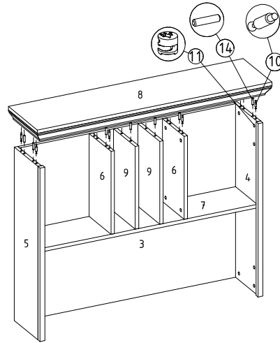
10) Sağ yan parça, sol yan parça ve arka parçaya üst parça montajı
