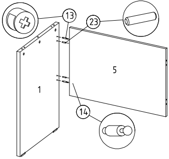
⑤ Yan parçaya arka perde montajı
