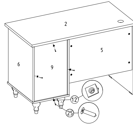
⑪ Arkalık sabitleyici montajı
