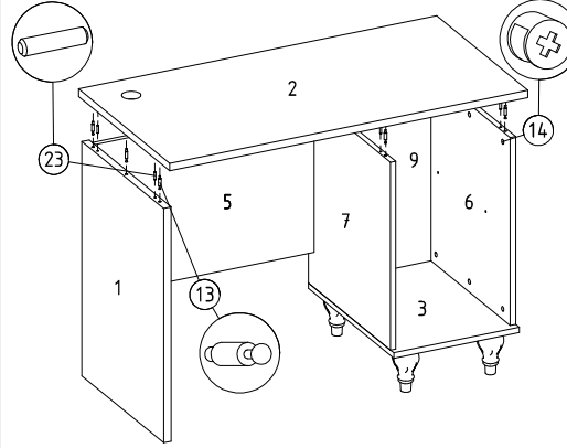
⑦ Üst tabla montajı
