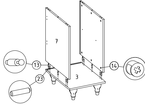
② Alt parçaya sağ yan parça ve sol yan parça montajı
