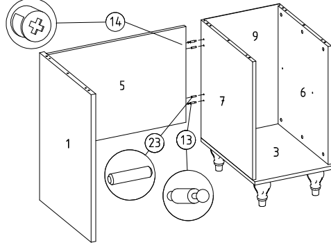
⑥ Sol yan parçaya arka perde montajı
