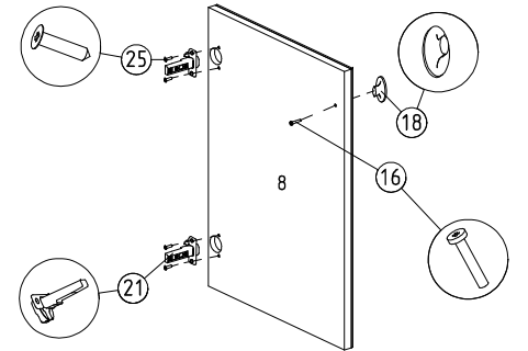
⑫ Mentеше ve kulp montajı
