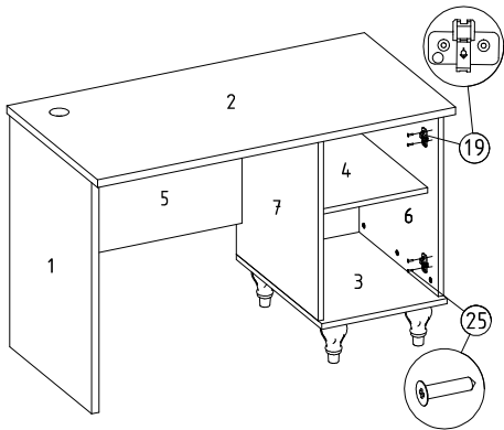
⑨ Mentеше tabanı montajı
