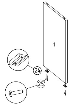
⑧ Raf pimi montajı
