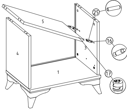
⑦ Sağ yan parça ve sol yan parçaya üst parça montajı
