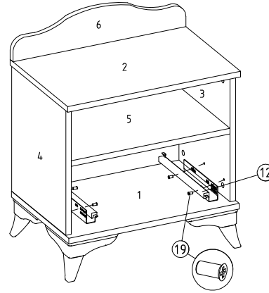
⑧ Sağ yan parça ve sol yan parçaya ray montajı
