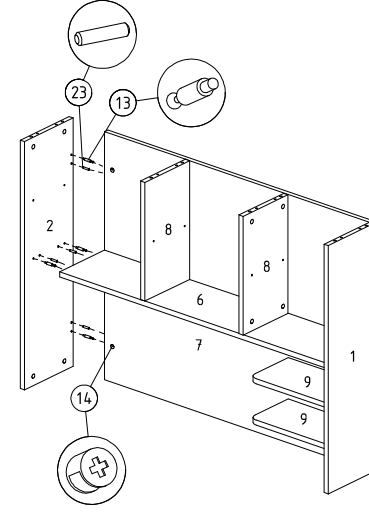
7 Arka parça, sabit raf ve seyyar rafa sol yan parça montajı
