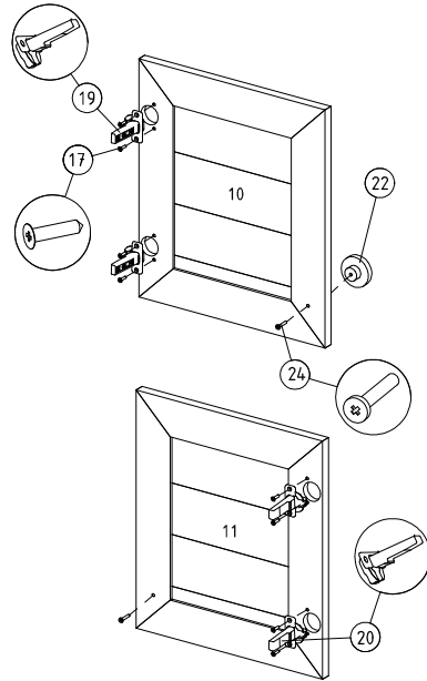
10 Kapaklara menteşe ve kulp montajı
