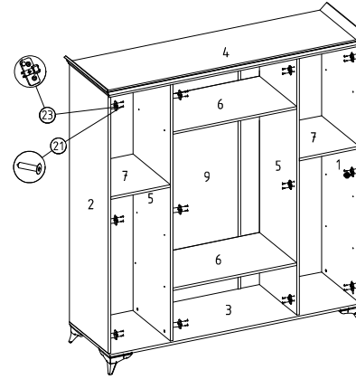
⑬ Tapa minifix montajı
