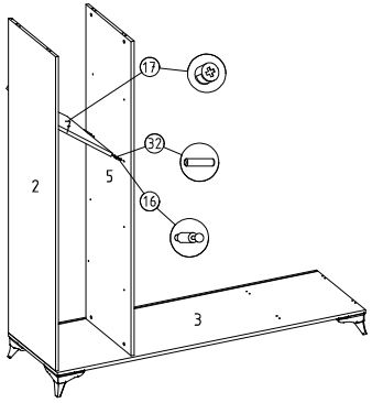
③ Sol yan parça ve orta dikmeye kısa bölme montajı
