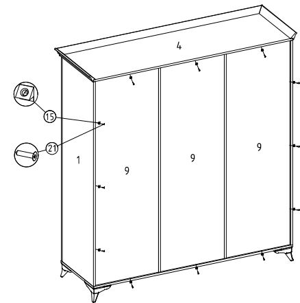
⑭ Arkalık sabitleyici montajı
