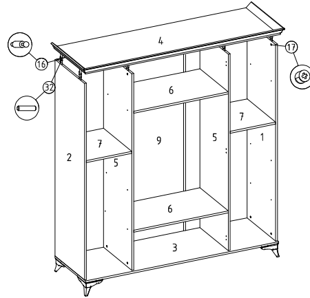
⑫ Askı flanşı montajı
