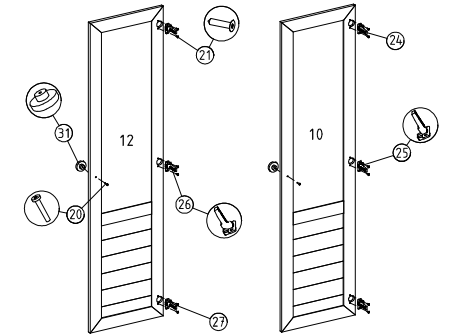
⑭ Arkalık sabitleyici montajı
