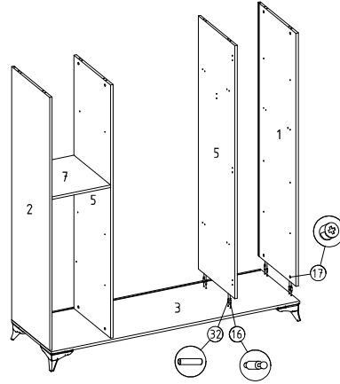
⑧ Sağ yan parça, sol yan parça ve orta dikme üst parça montajı
